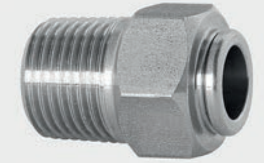
3/8" boru için paslanmaz 3/8" erkek bağlantı 303 kalite NPT
