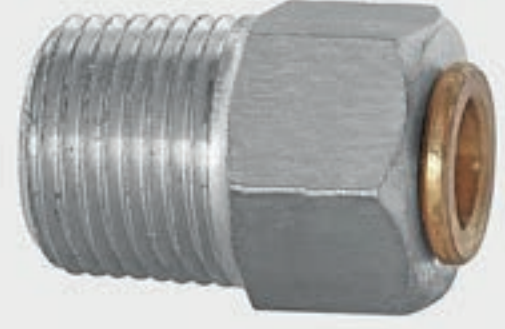
5/16" boru için 3/8" erkek bağlantı NPT
